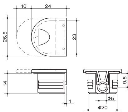
寸法図
