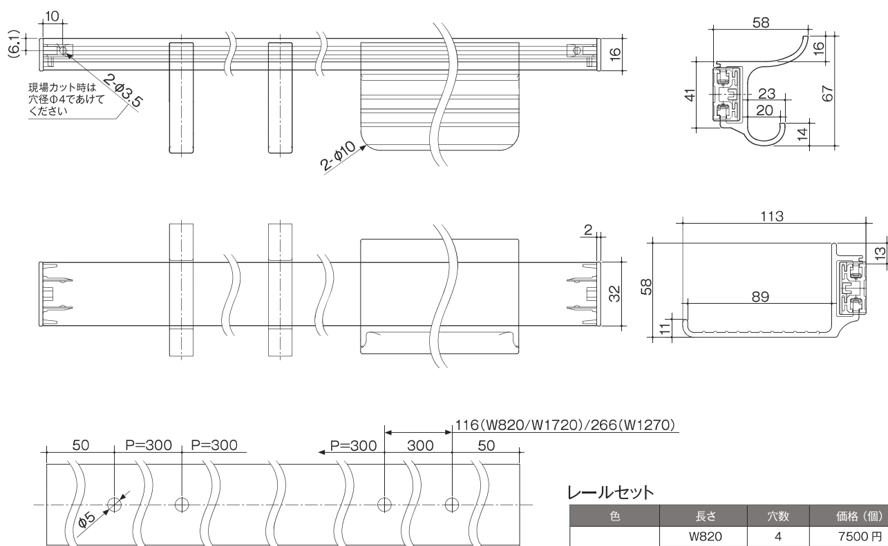
納まり図
