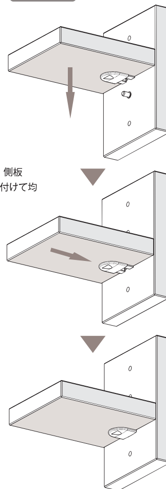
取付図
