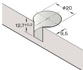
加工図
