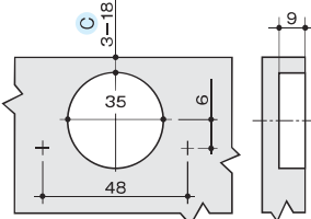
加工図
