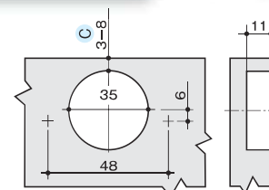
加工図
