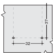
加工図
