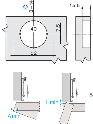
加工図
