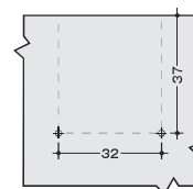
加工図
