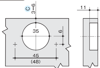
加工図
