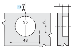
加工図
