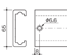
穴加工図
