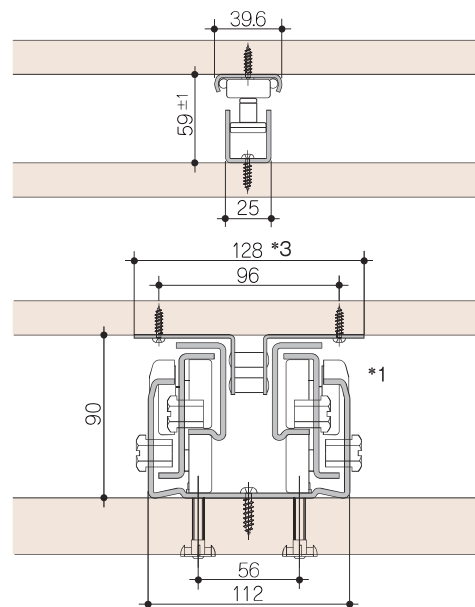
取付図
