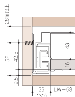
取付寸法図 H63
