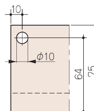
側板 89mm の場合
