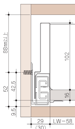
取付寸法図 H186
