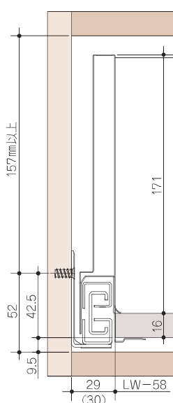
取付寸法図 H186
