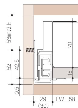
取付寸法図 H90
