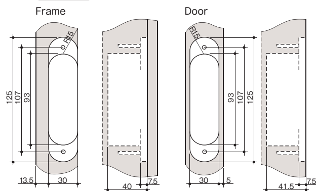
加工図
