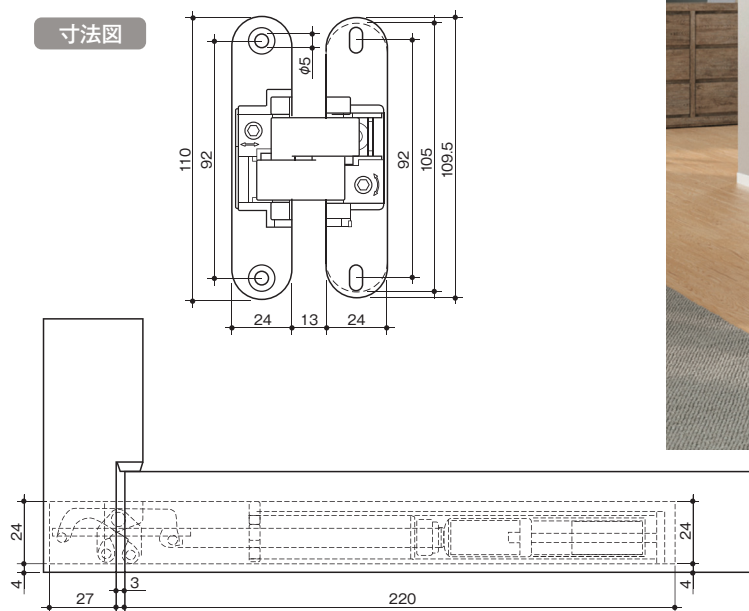
加工図
