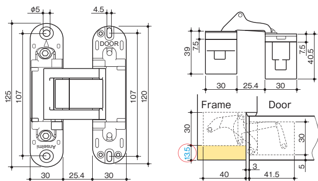
寸法図
