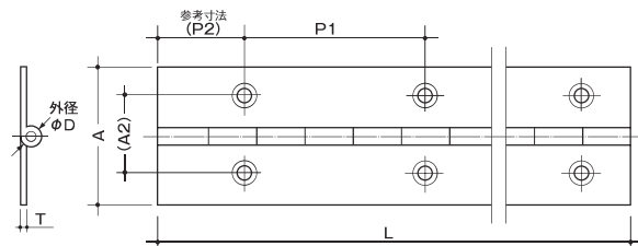
寸法図
