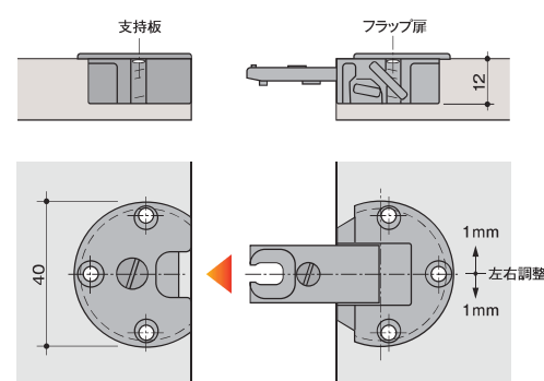
取付方法
