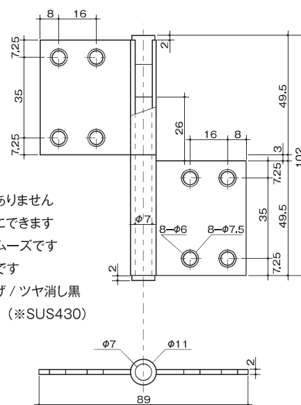
寸法図
