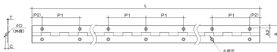
寸法図
