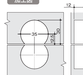
加工図
