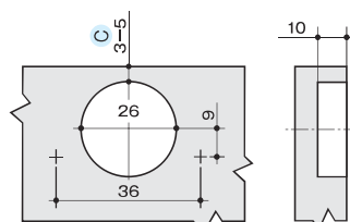
加工図
