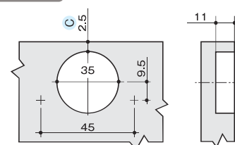
加工図
