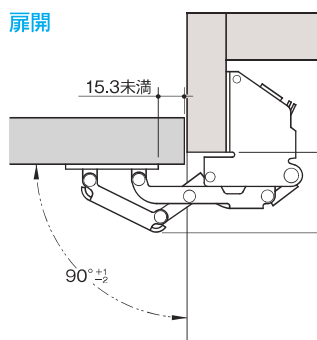
扉開
