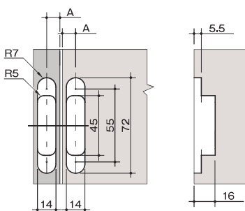
加工図
