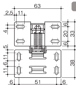
扉開
