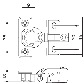
寸法図
