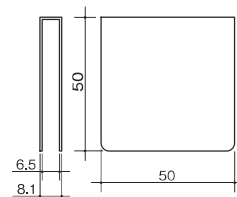
寸法図
