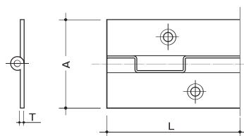
寸法図
