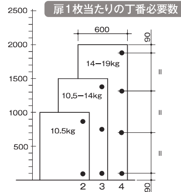
扉 1 枚当たりの丁番必要数
