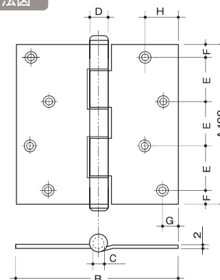
寸法図
