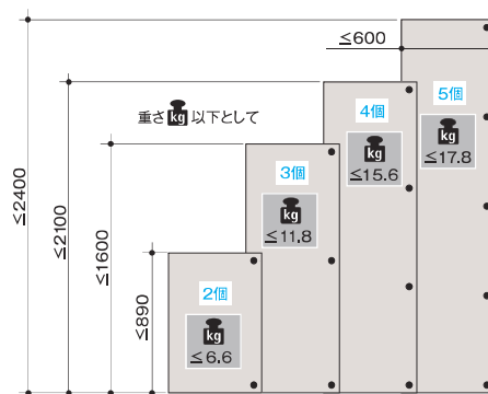
扉高さ・扉重量に対する個数の目安
