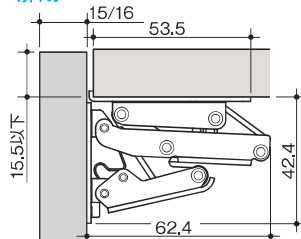
扉閉
