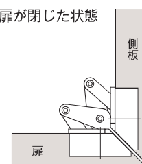
取付図
