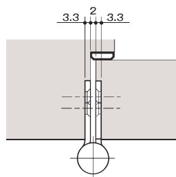
取付図
