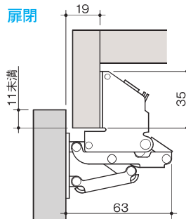
扉閉
