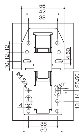
寸法図
