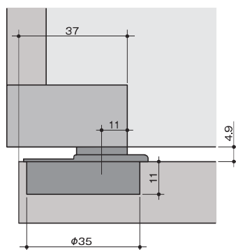
寸法図
