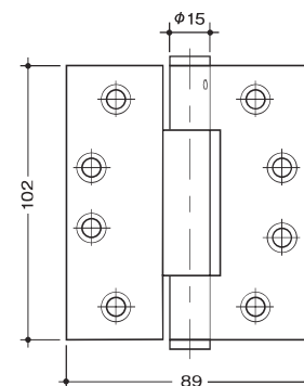
寸法図
