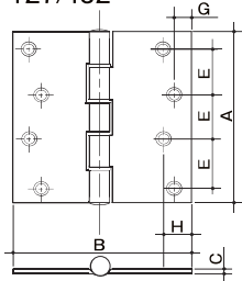
寸法図
