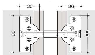
寸法図
