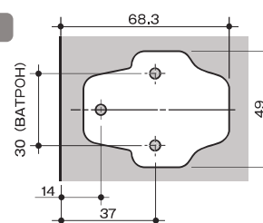
加工図
