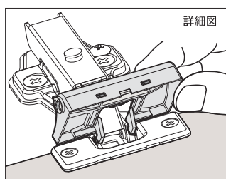
取付け方法
