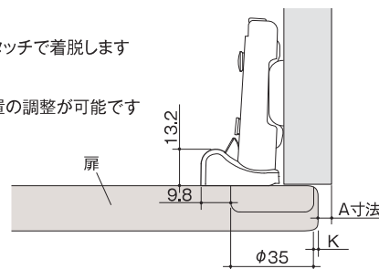
加工寸法図
