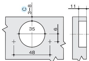
加工図
