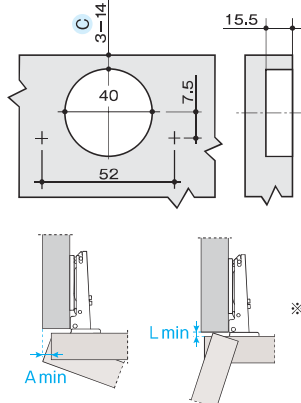
加工図
