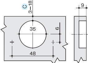
加工図
