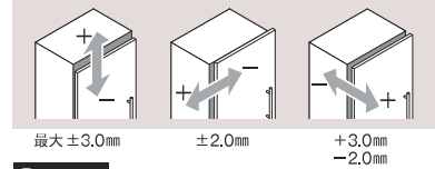
加工図
