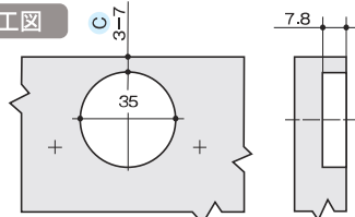
加工図
