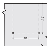
加工図
