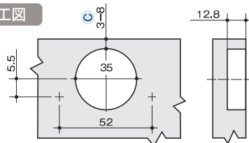
加工図
