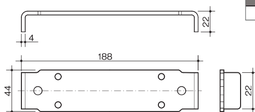
寸法図
