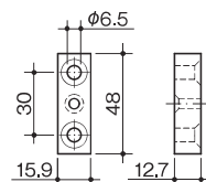
寸法図
