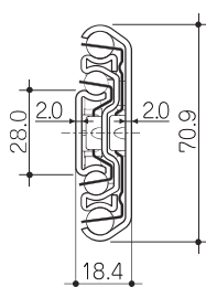
断面図
