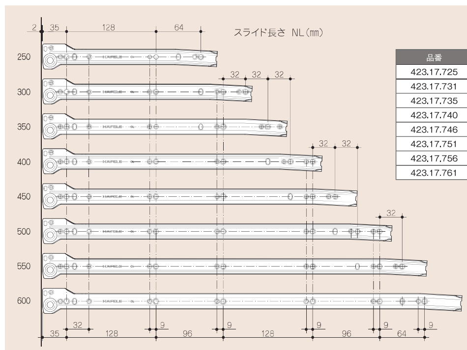
受けレールネジ穴位置
