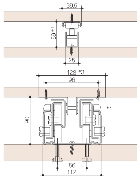
取付図
