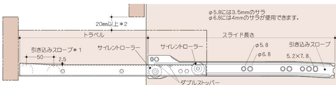
受けレールネジ穴位置
