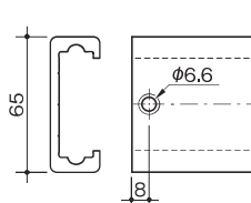
穴加工図
