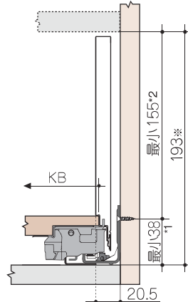
C 側板高さ：177 mm
