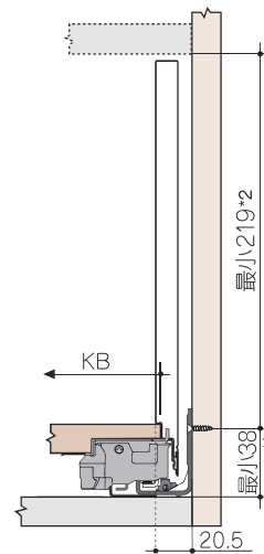
F 側板高さ：241 mm
