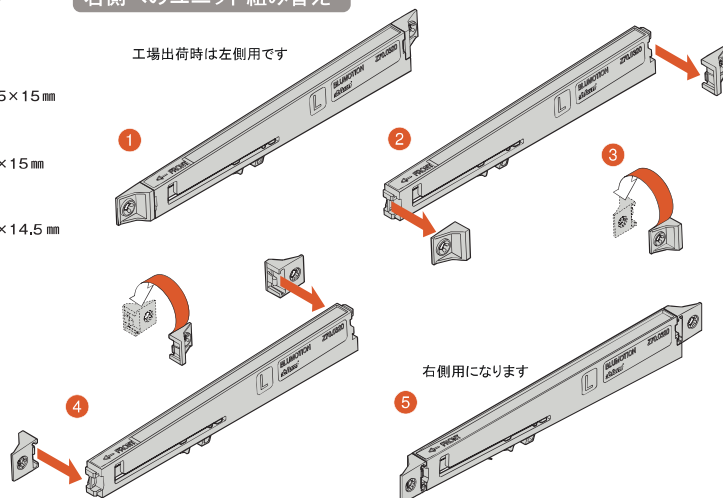
右側へのユニット組み替え
