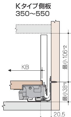
K 側板高さ：128.3 mm
