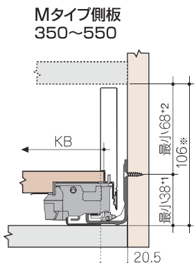
M 側板高さ：90.5 mm
