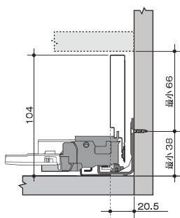
キャビネット最小寸法
