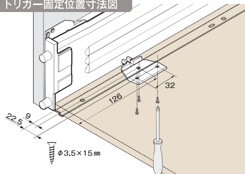
トリガー固定位置寸法図
