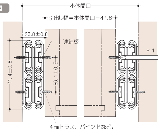
取付図
