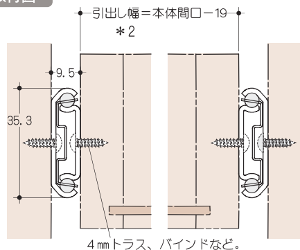
取付図
