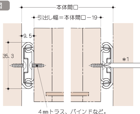
取付図
