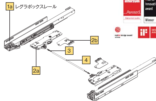
モベント・レグラボックスレール用 チップオンブルモーションユニット本体・ラッチ 左/右
