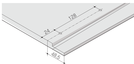
16mm厚パーティの場合の切断寸法
