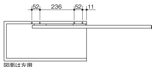
図面は左用
