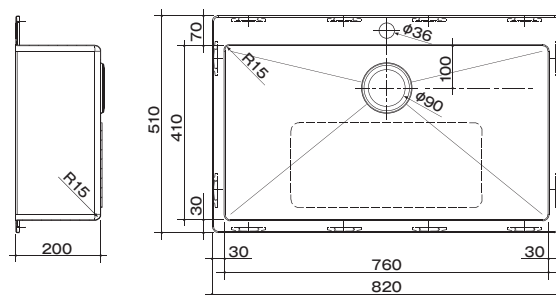
寸法図
