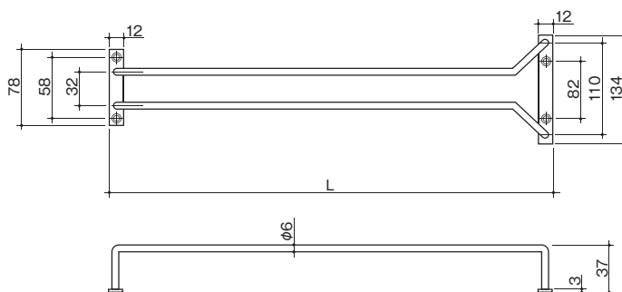
寸法図
