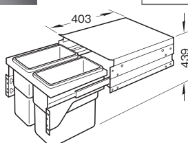
寸法図
