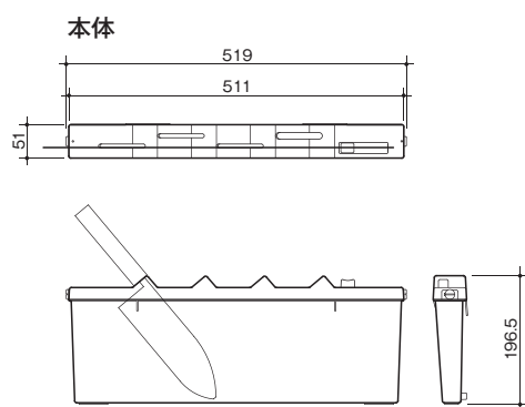
取付図
