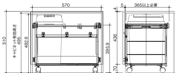
図は 503.72.506 (キャビネット幅 600 mm用)
