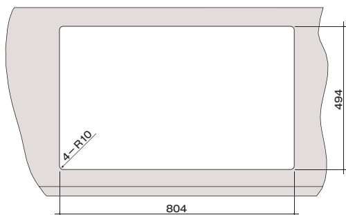
加工図
