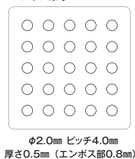
エンボス原寸
