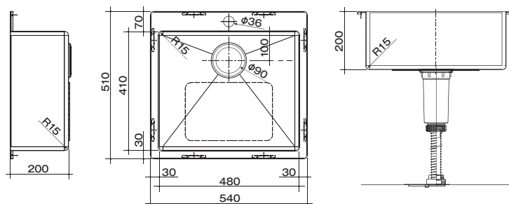
寸法図
