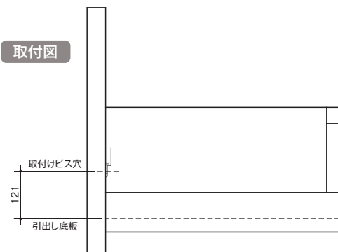
マルチボックス
