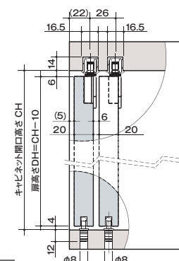
取付寸法図
