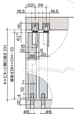
取付寸法図
