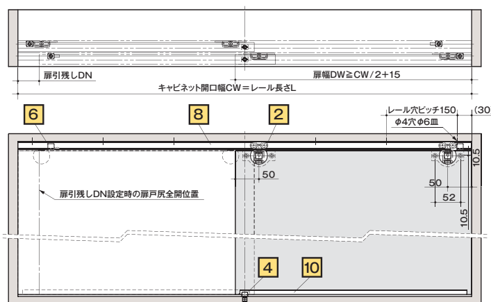
取付寸法図
