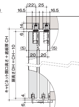
取付寸法図
