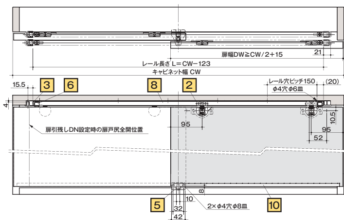
取付寸法図
