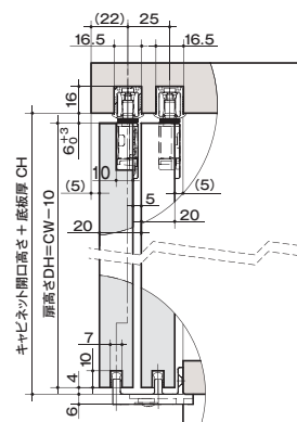
取付寸法図
