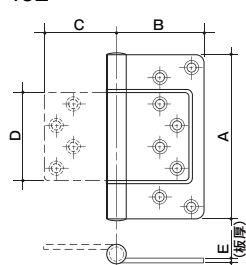
寸法図
