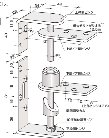
名称・寸法図
