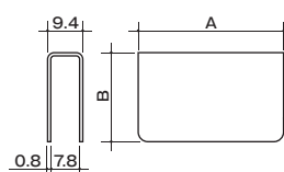
寸法図
