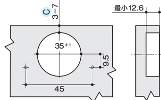
加工図
