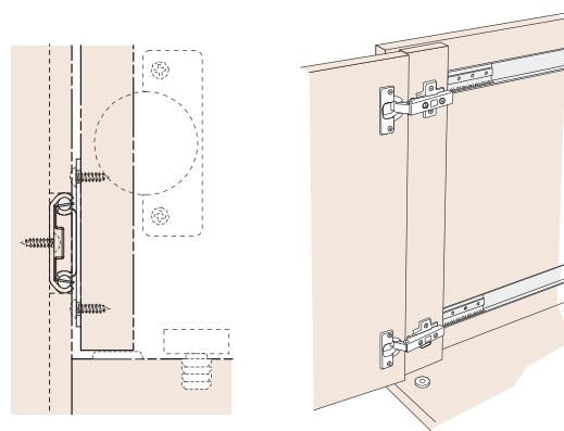
取付図
