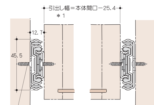
取付図
