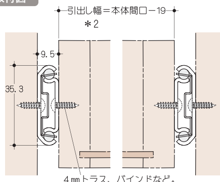
取付図
