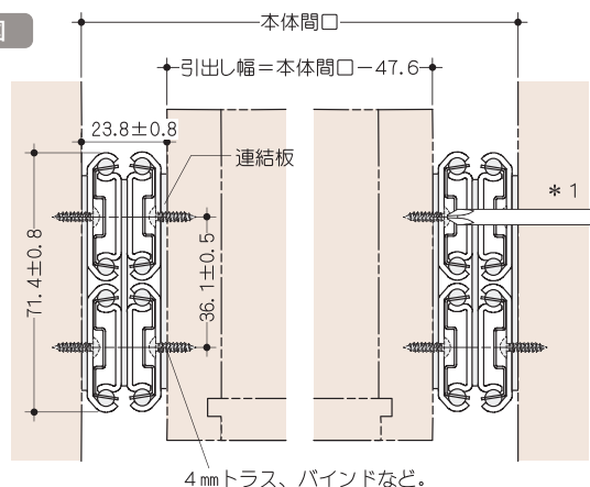
取付図
