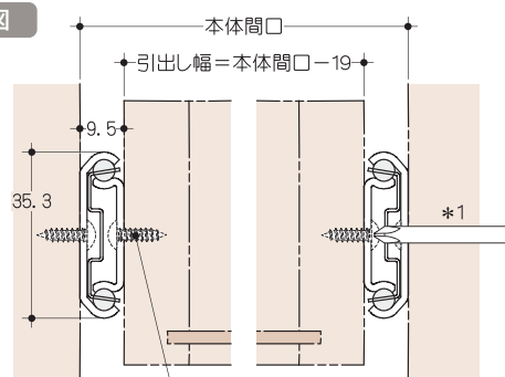
取付図
