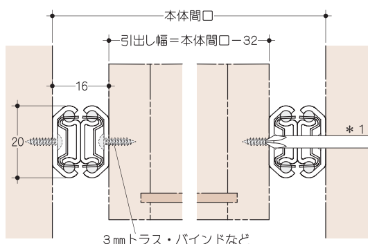
取付図
