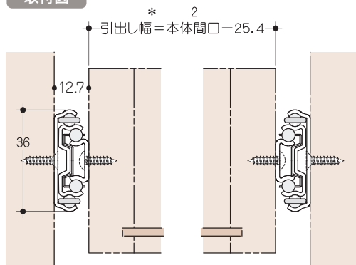
取付図
