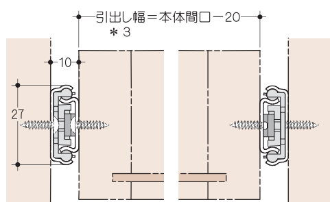
取付図
