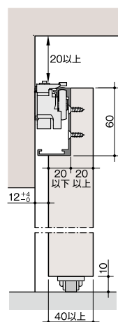
固い床材の場合の下部ガイド
