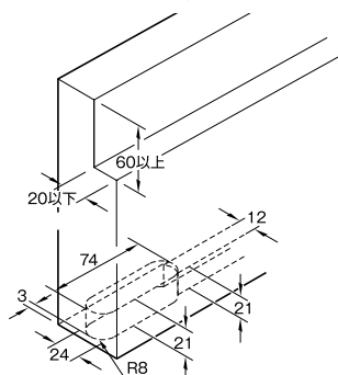
エンドキャップあり
