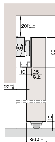
柔らかい床材の場合の下部ガイドと床レール
