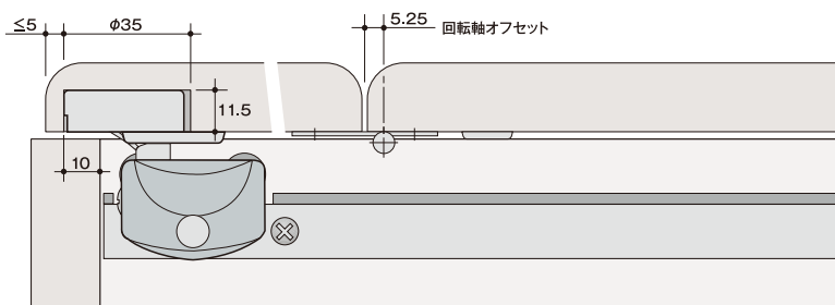
金具取付図
