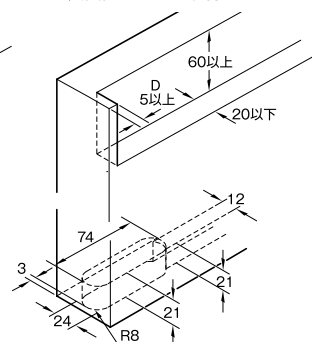
裏面隠しレール取付
