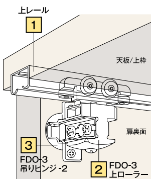
1 FDO-3 上レール (ステンレス色) アウトセットタイプの上レール L=2m
