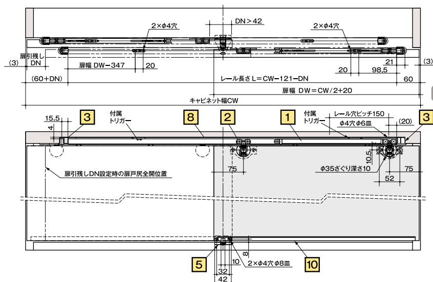
取付寸法図
