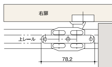
取付寸法図
