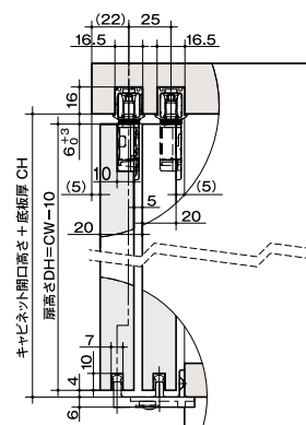
取付寸法図
