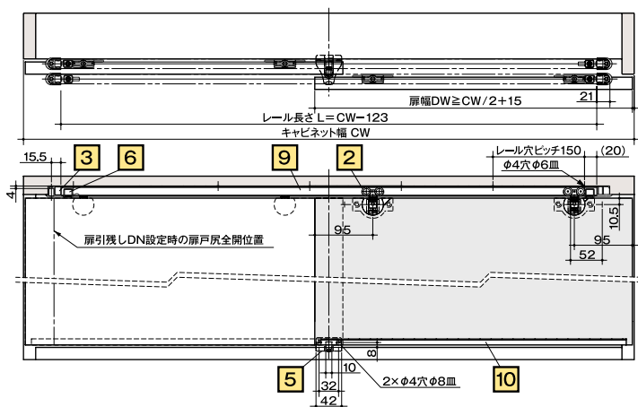
取付寸法図
