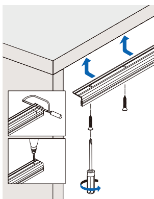
レール取付図
