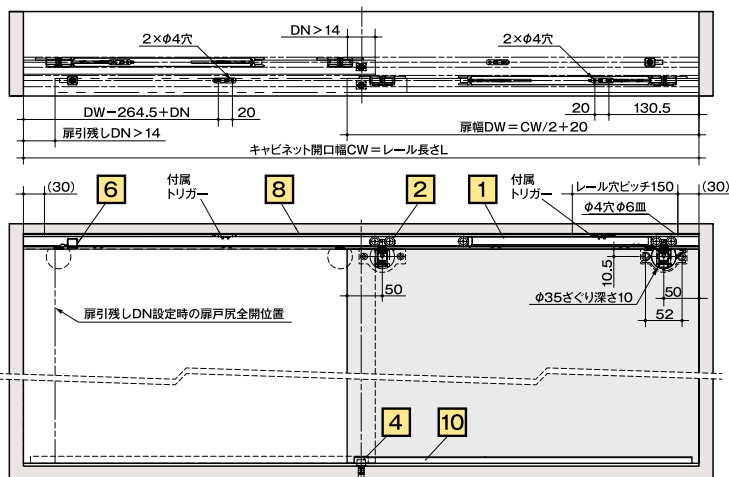
取付寸法図
