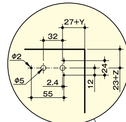
穴加工図
