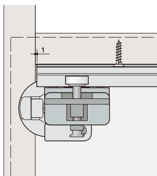
納まり図・寸法図
