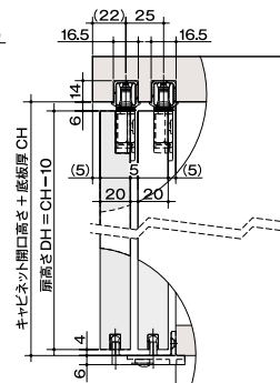
取付寸法図
