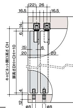
取付寸法図
