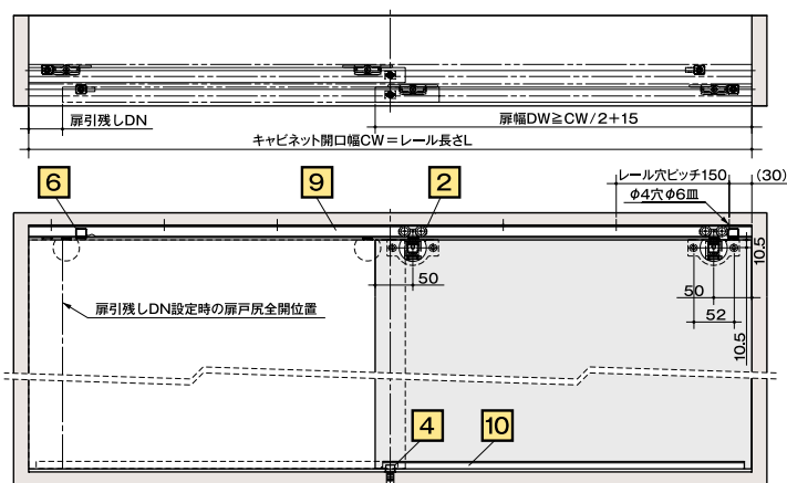
取付寸法図
