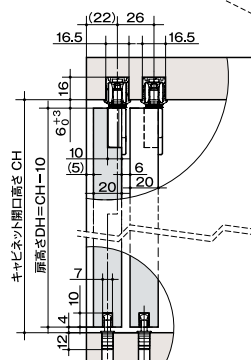
取付寸法図
