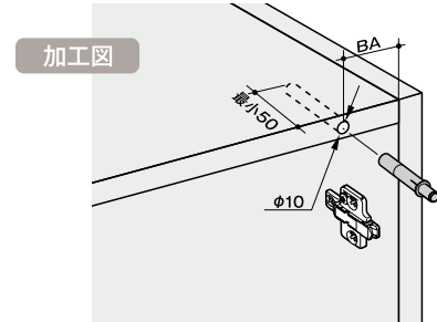
標準キャビネット 取付位置 (BA)
