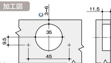
加工図
