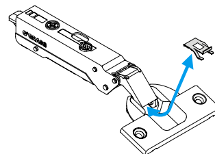
■ 85° 角度ストッパー取付図
