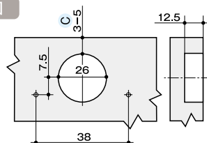
加工図
