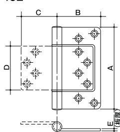
寸法図
