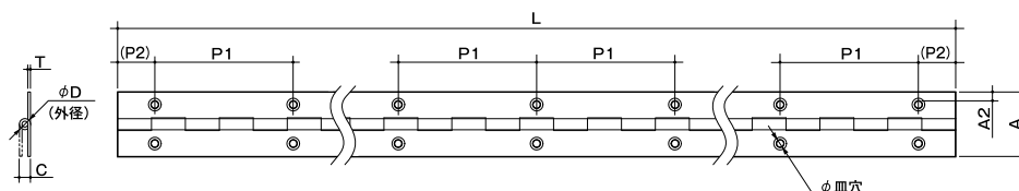
寸法図
