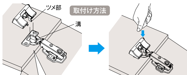
詳細図
