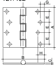
寸法図
