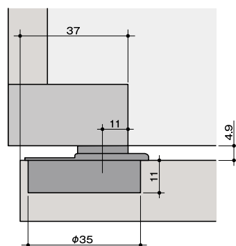
寸法図
