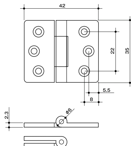
寸法図
