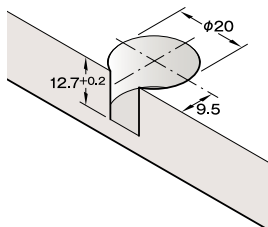
加工図
