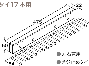
寸法図
