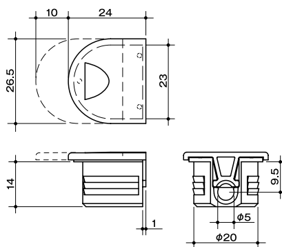
寸法図
