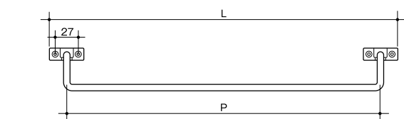
寸法図
