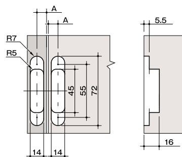
加工図
