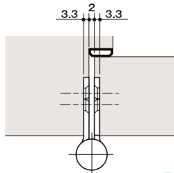
取付図
