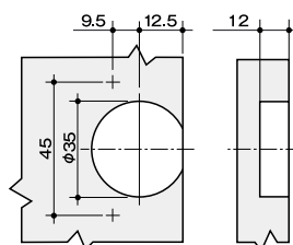
寸法図
