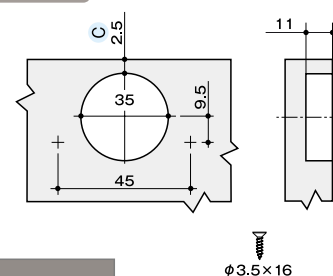
加工図
