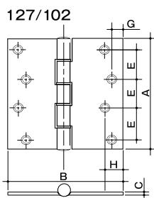
寸法図
