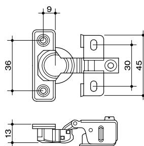
寸法図
