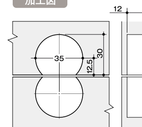
加工図
