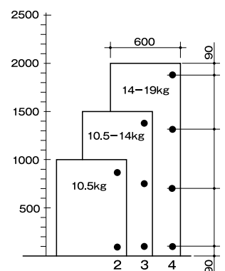
扉1枚当たりの丁番必要数
