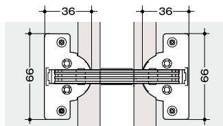
寸法図
