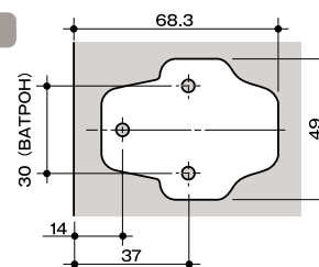
加工図
