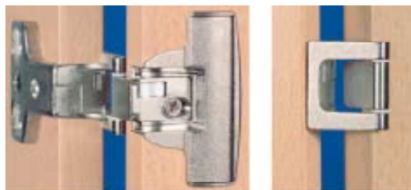
薄型ヒンジでキャビネット内部を利用
