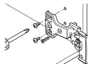
側板ヒンジの固定方法
