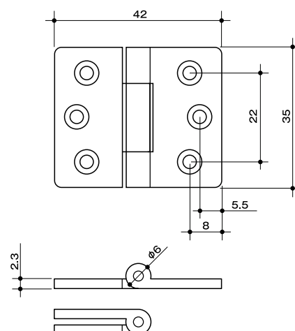
寸法図
