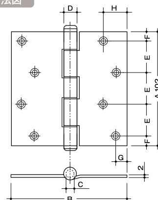
寸法図
