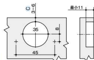
加工図
