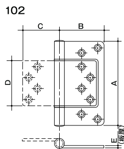
寸法図
