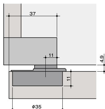
寸法図
