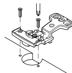
側板ヒンジの固定方法
