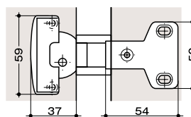
寸法図
