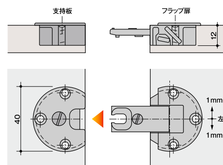
取付方法
