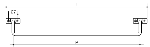
寸法図
