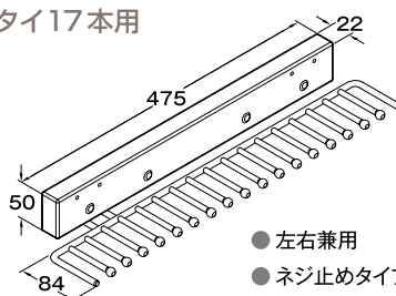
寸法図
