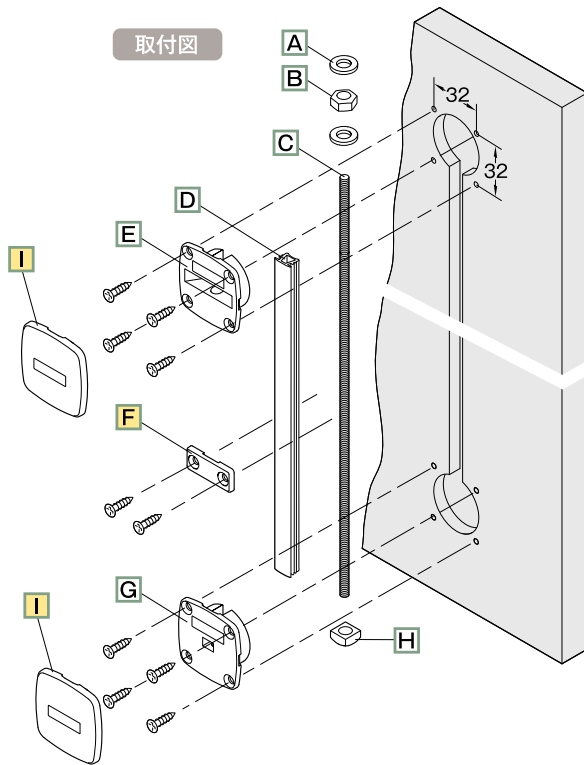
取付図
